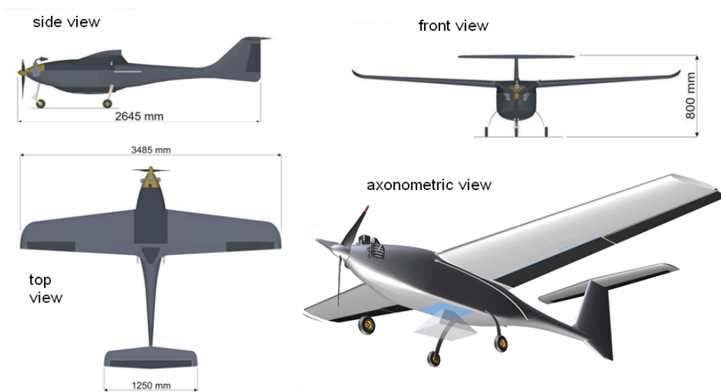
Fig. 4. Mini UAV.
